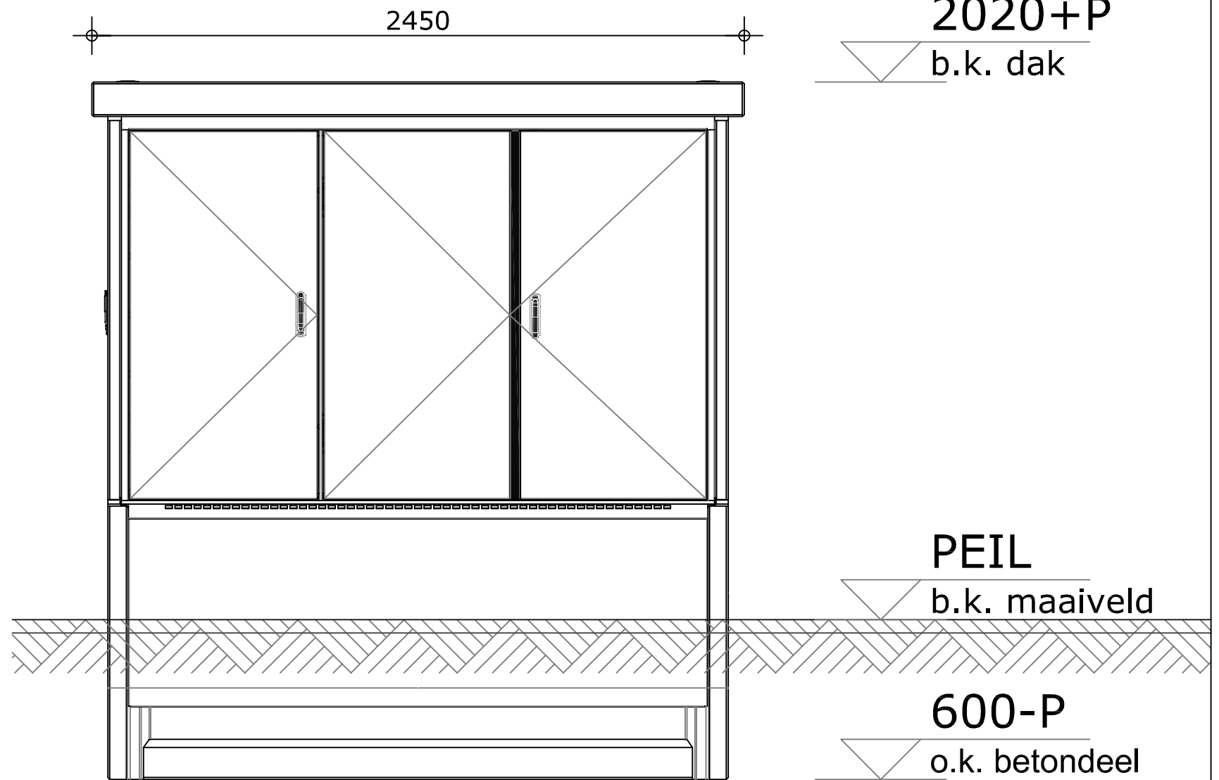
VOORAANZICHT
