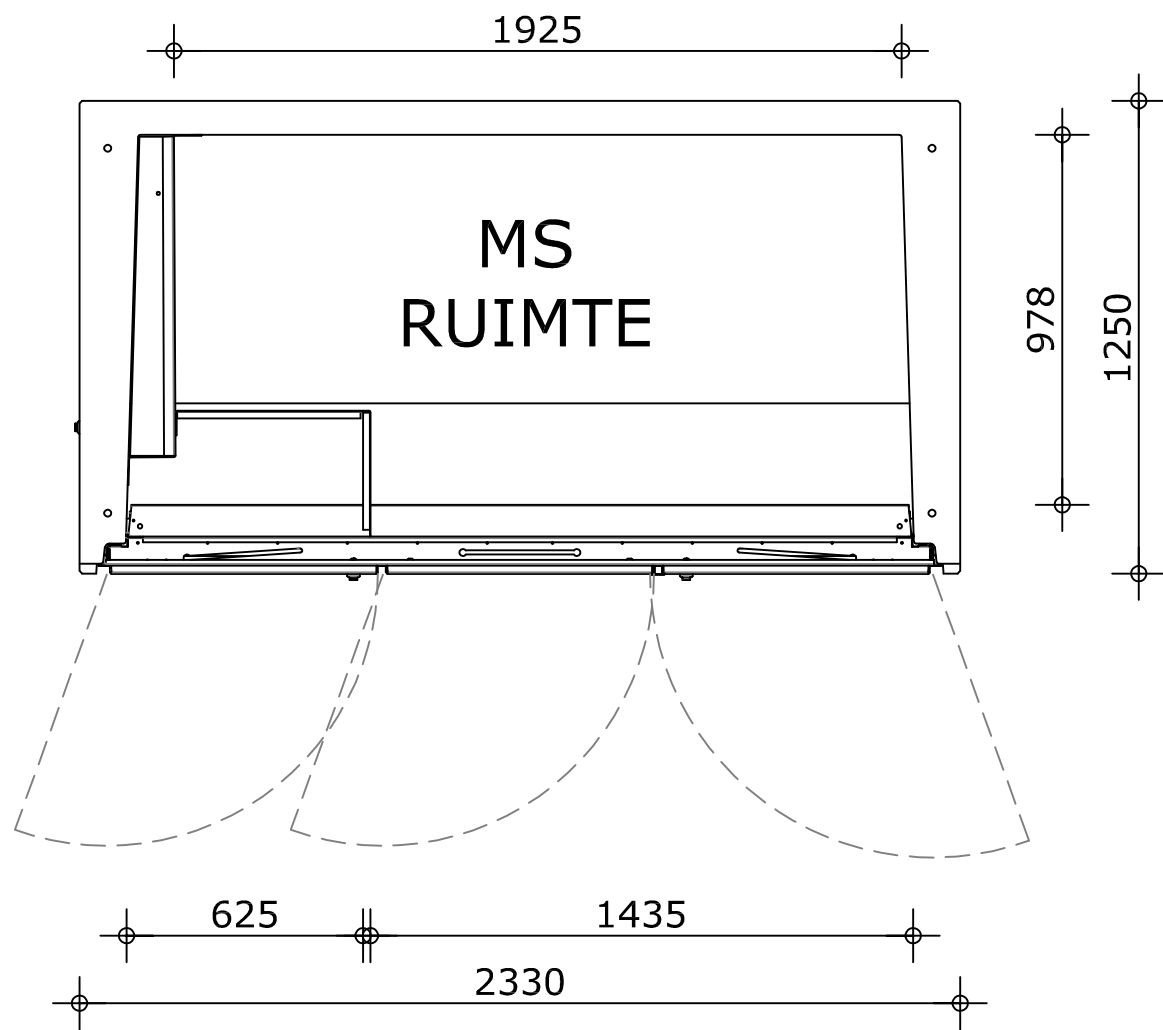
VLOERPLAN
